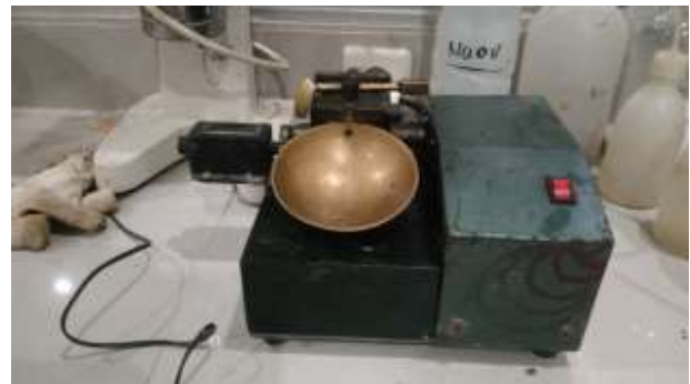
Alat uji batas batas konsistensi (cassagrande)
