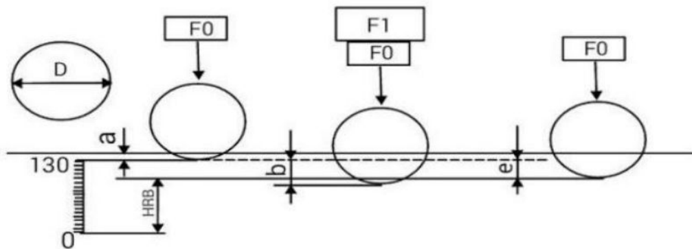
Pengujian kekerasan Rockwell dengan indenter bola
