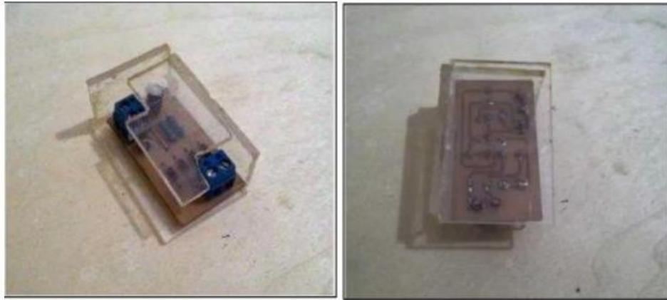
Gambar 2. 8 Tampak atas (kiri) dan bawah (kanan) rangkaian penyearah dan regulator (Akmal, 2017)
