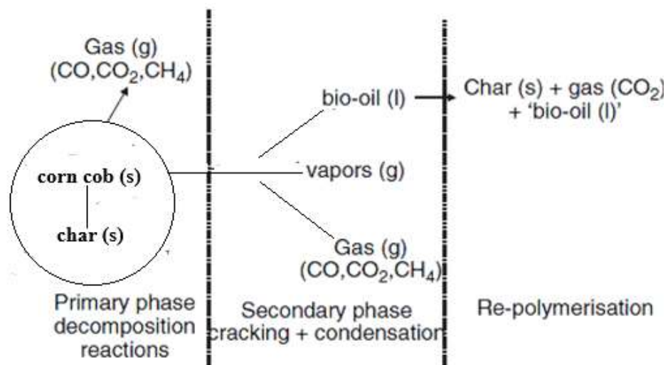
Gambar 3. Representasi Jalur Reaksi Pirolisis Bonggol Jagung
