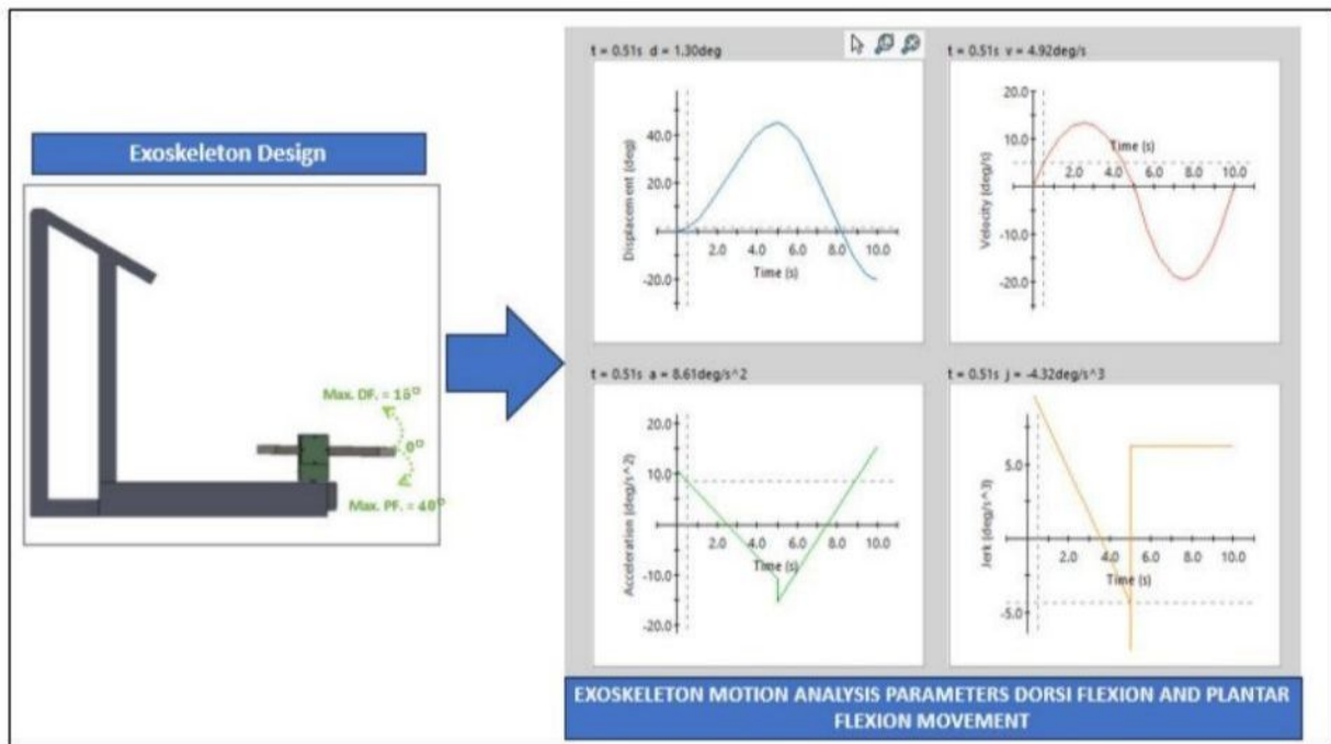
Gambar 4. 6 Simulasi gerakan pada desain eksoskeleton dengan kecepatan lintasan sudut Gerakan dorsiflexi/fleksi plantar \omega = 40^{\circ}/s ( 0.698 \text{ rad/s} ).
